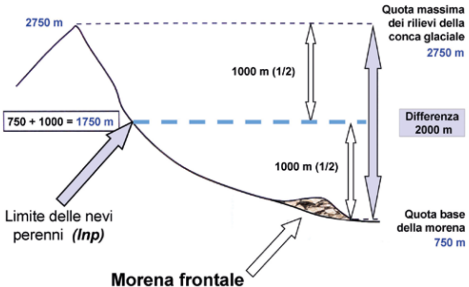
Fig. 39 Schematizzazione dei calcoli finalizzati al recupero del limite delle nevi perenni ( lnp ), valutato per una data morena frontale. Il metodo vale per ghiacciai di limitate estensioni.
