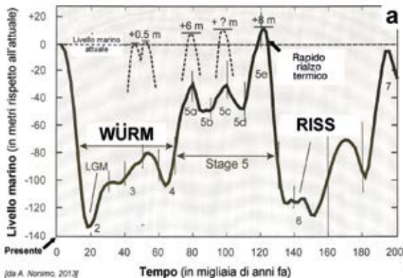
Fig. 36 Il Tardo-glaciale würmiano: il "colpo di coda" della glaciazione würmiana. (a: da Martinson et al., 1987 modif.).
