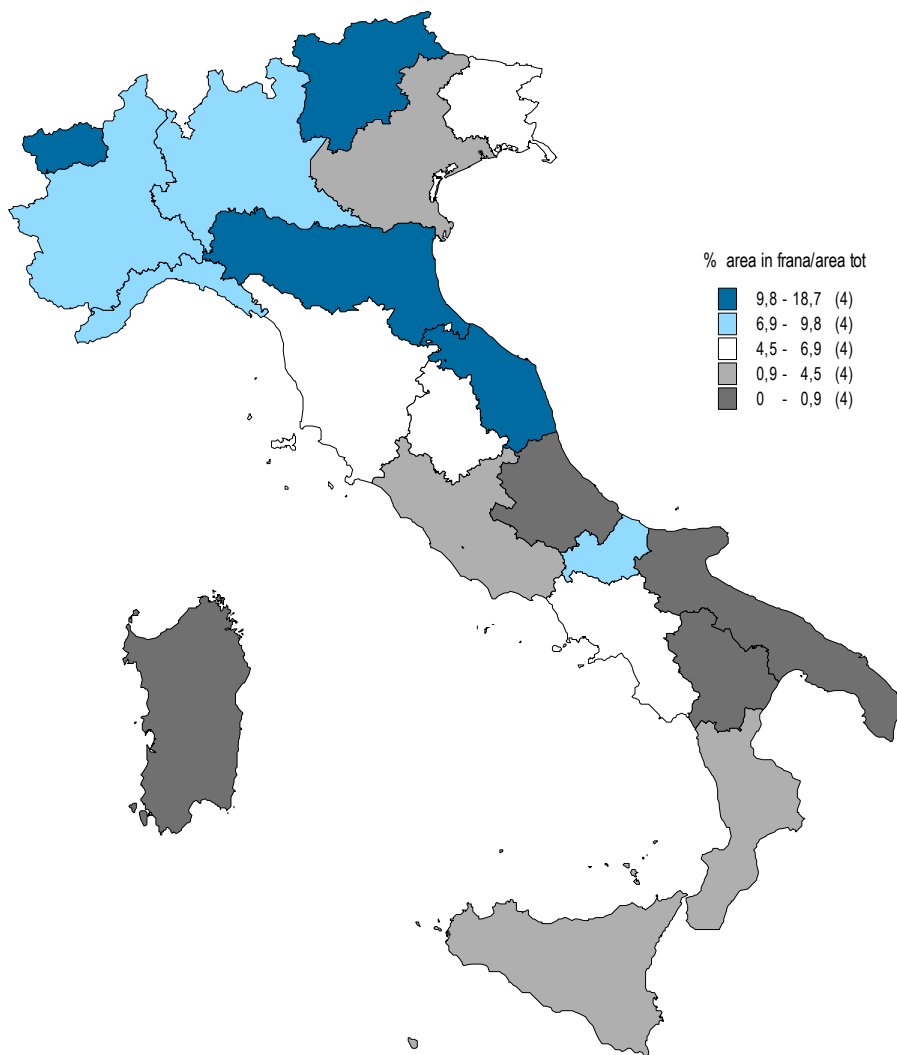
Cart. 3.1 – ITALIA INDICE DI FRANOSITA'– Anno 2005
